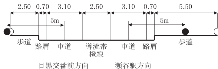
図 9.3-3(6) 道路断面及び基準点の位置 (No. 6)
