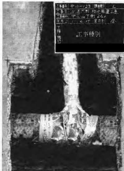
分岐下部状況写真 (サドル状付分水栓穿孔工事)
