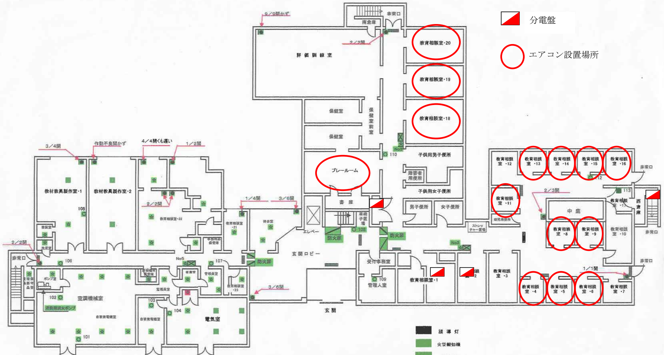
一階平面図
