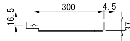
側面図
