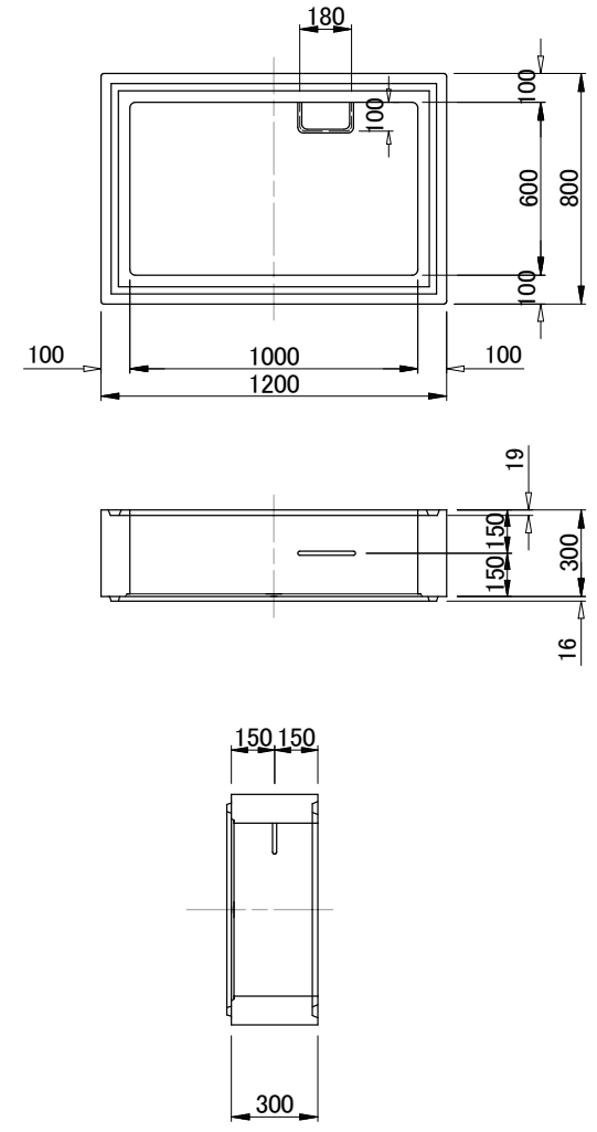
Dブロック構造図
