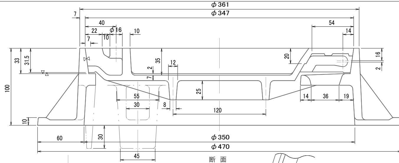
断面
