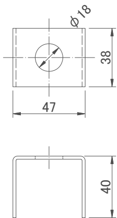
回り止め金具詳細図
