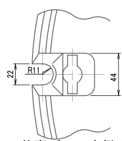
蓋裏パール穴鍵穴部詳細
