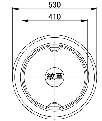
ふた 縁塊
