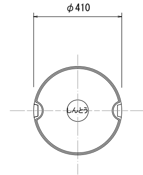
ふた
