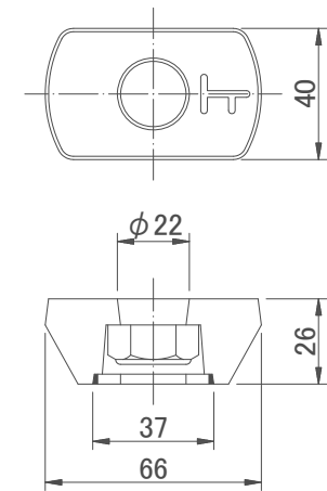
ゴムパッキン詳細図
