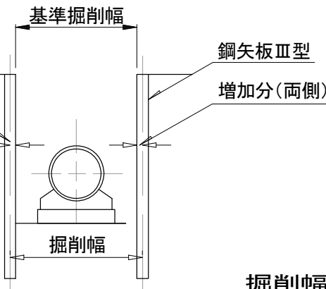
(4) 鋼矢板 III 型
