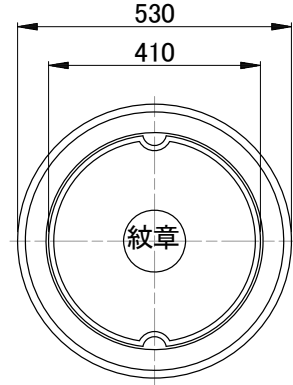
ふた 縁塊
