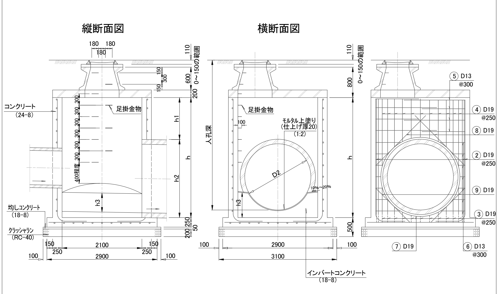
第5種人孔構造図(1)
