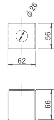
回り止め金具詳細図
