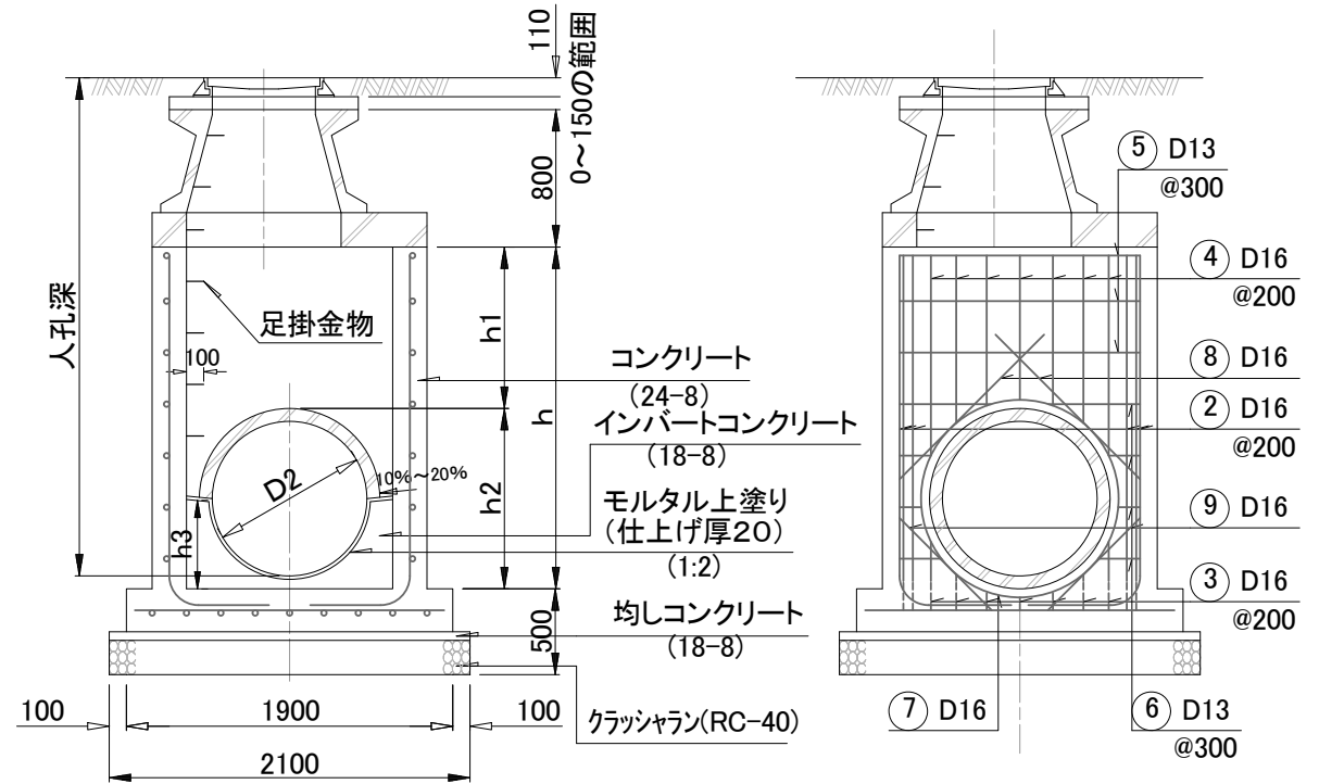
横断面図
