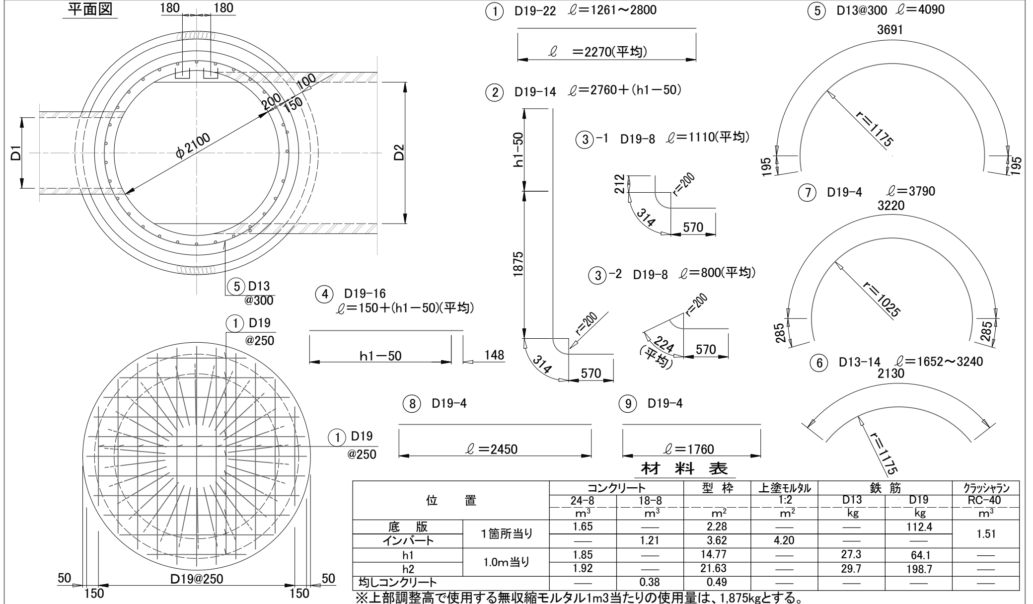
第5種人孔構造図(2)
