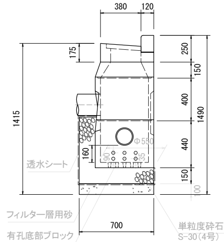
C-C 断面図
