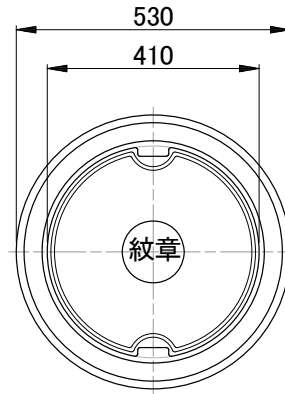
ふた縁塊
