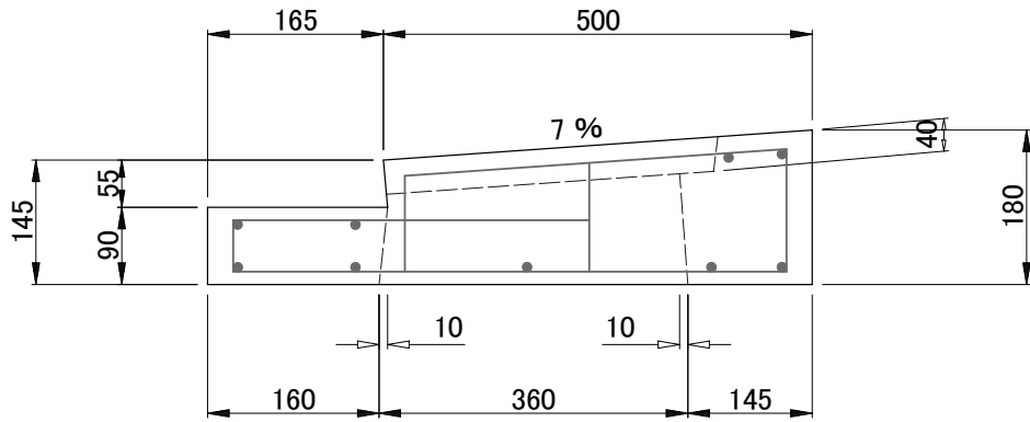
側面図
