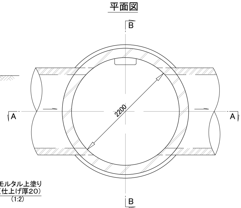
踊り場直壁
