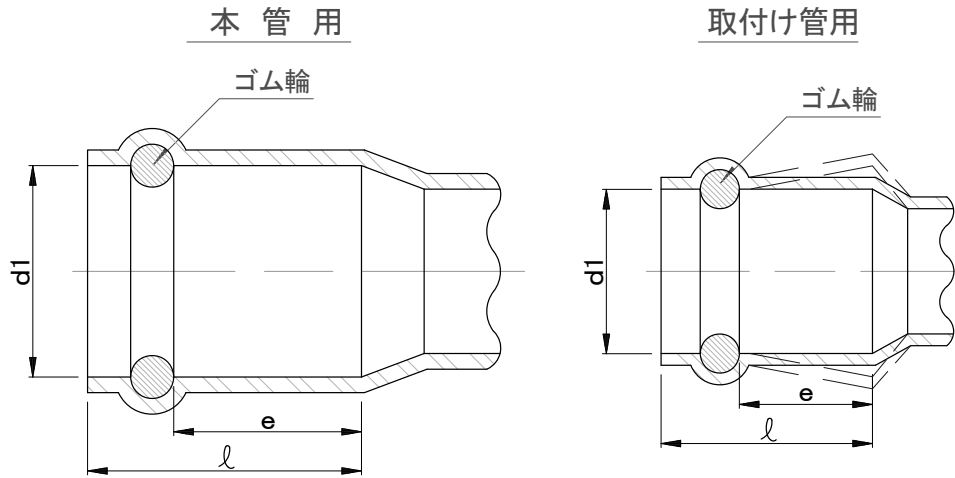
ゴム輪受口共通寸法表
