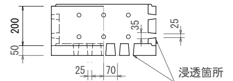
有穴底塊
