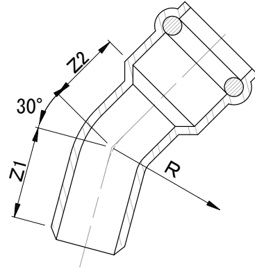
ゴム輪受口(略号30SR)
