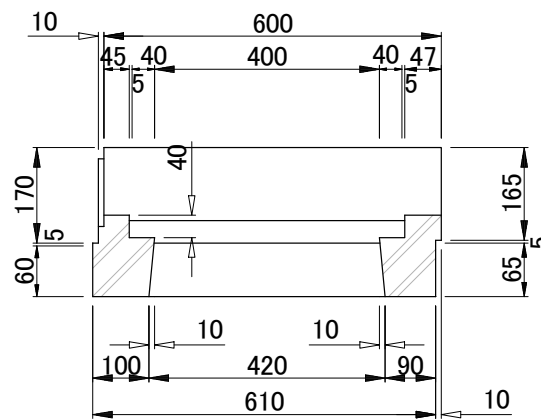
A-A断面図
