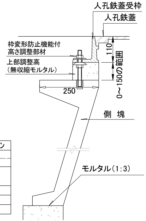
人孔蓋枠据付参考図
