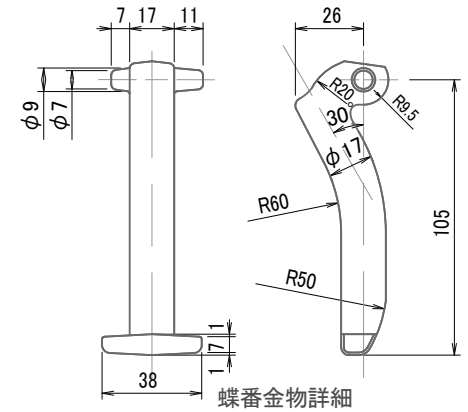
蝶番金物詳細
