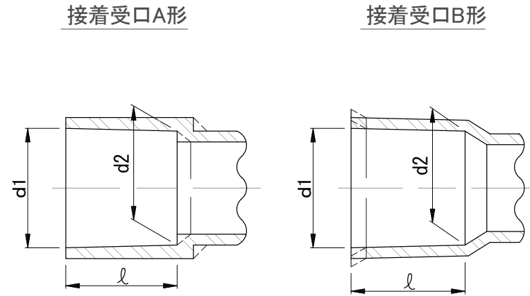
接着受口共通寸法表
