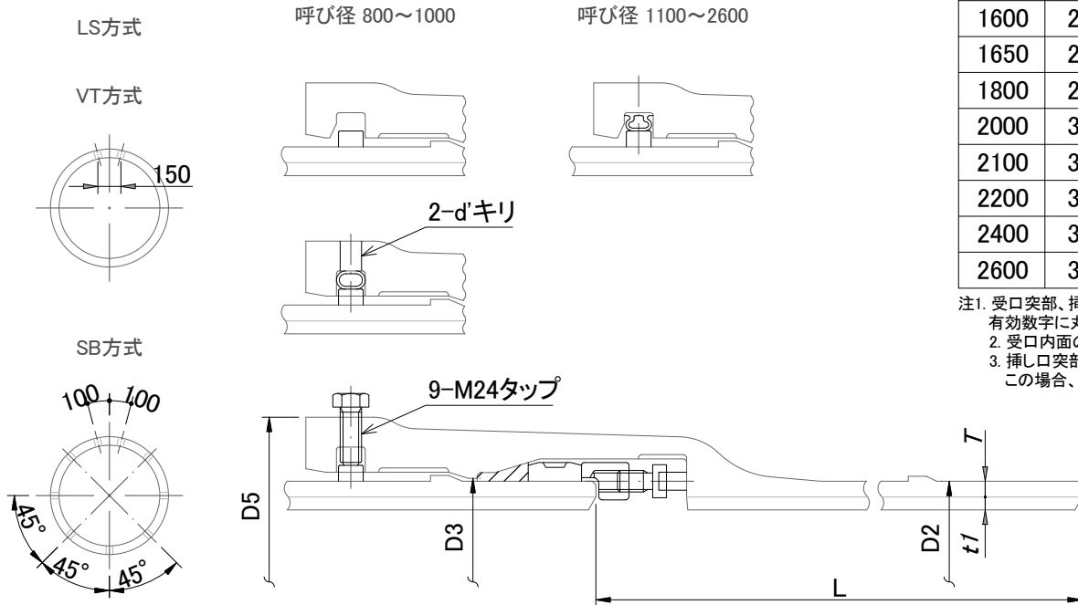
接合部詳細
