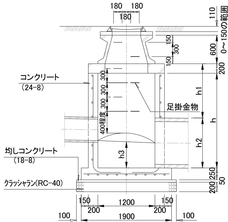
縦断面図
