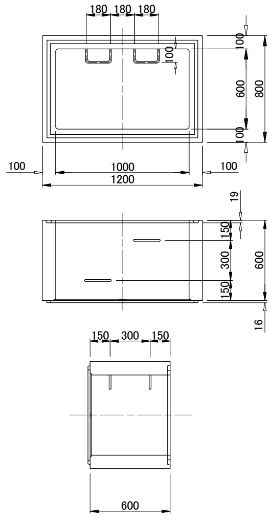
Cブロック構造図
