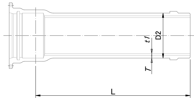
接合部詳細
