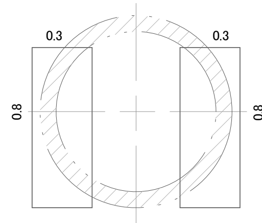
内径 800mm
