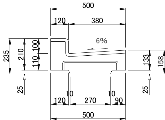
正面図
