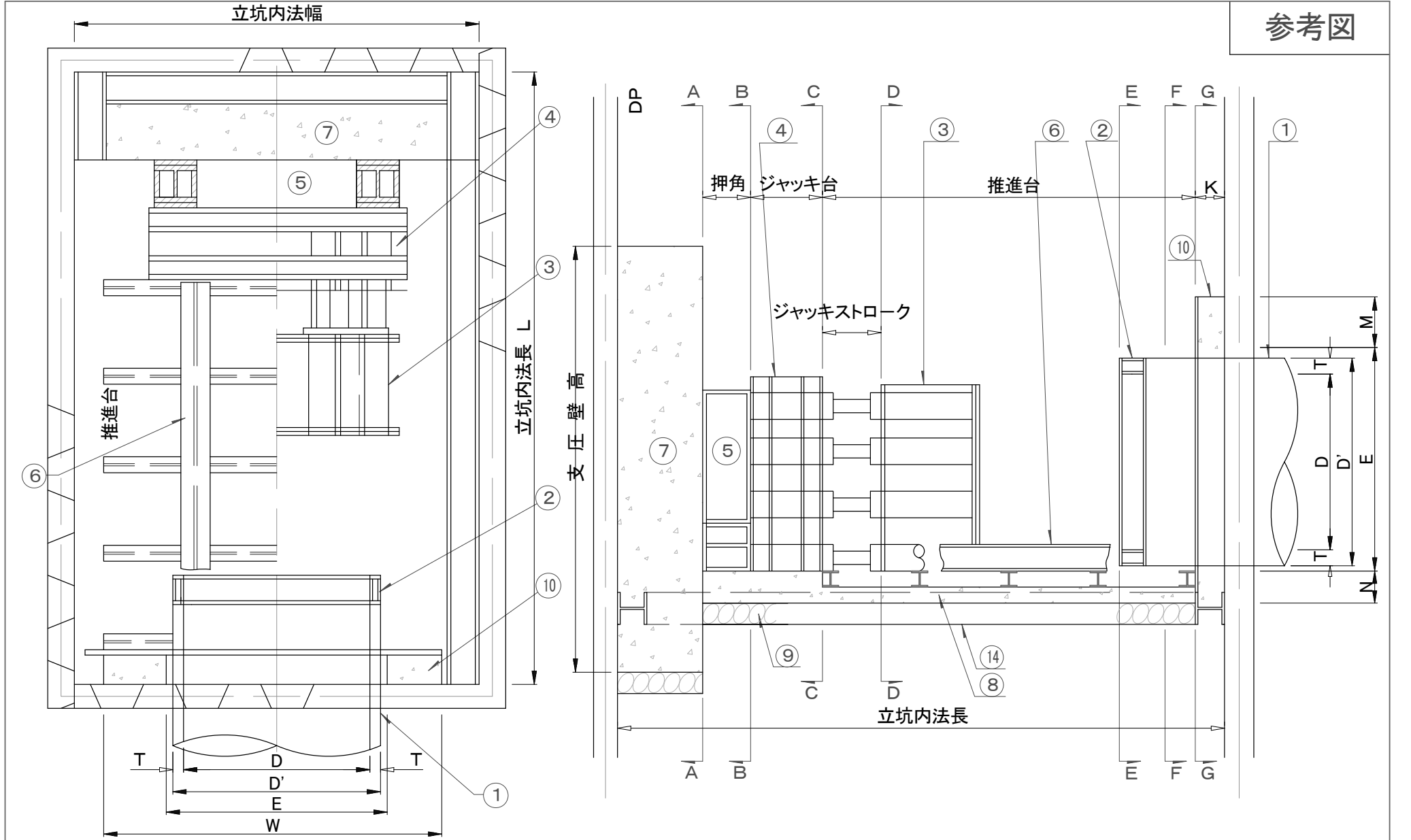
推進設備図(1)
