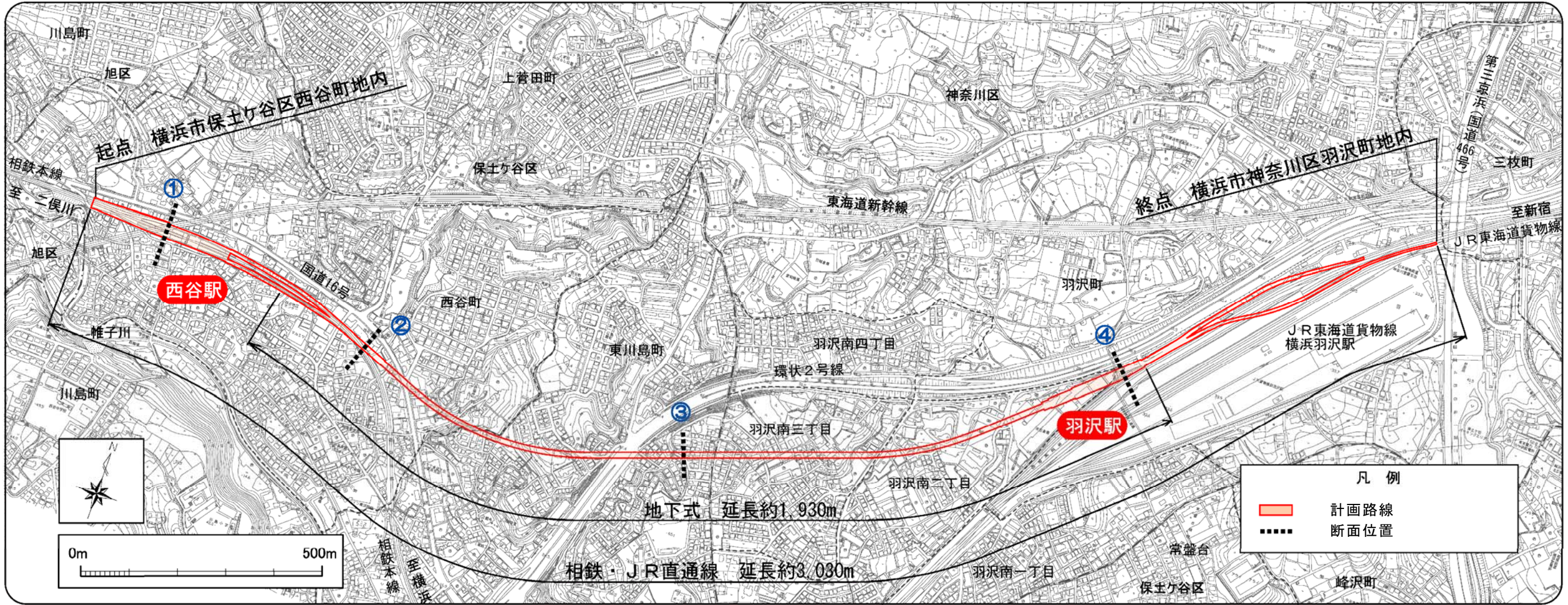
図 1-1(1) 平面図
