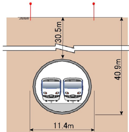
図 1-2 (3) 円形トンネル概略断面図 (③)
