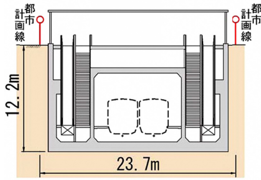
図 1.5-1(1) 羽沢横浜国大駅部概略断面図① 図 1.5-1(2) 箱型トンネル概略断面図②
