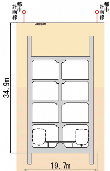
図 1.5-1(5) 新綱島駅部概略断面図⑤
