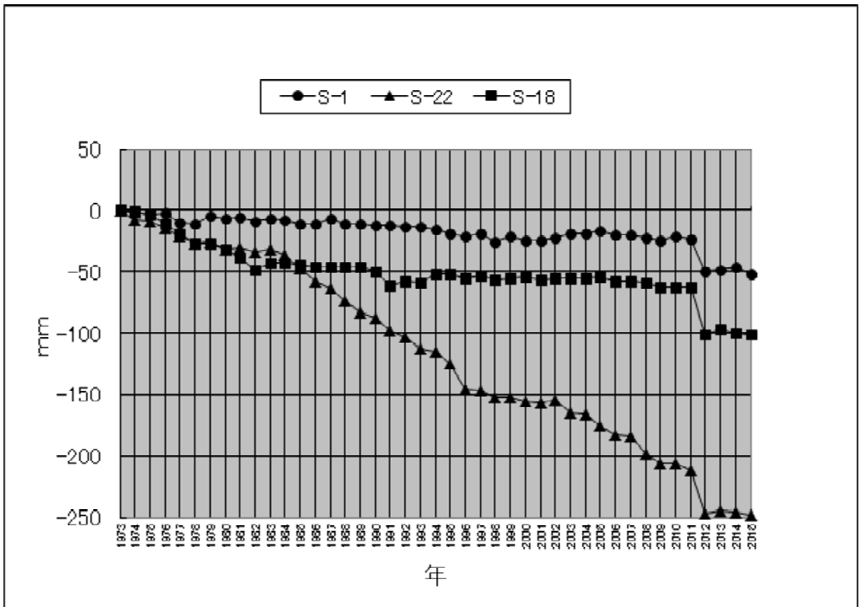
图 2-1-18 瀬谷区水准点经年变化
