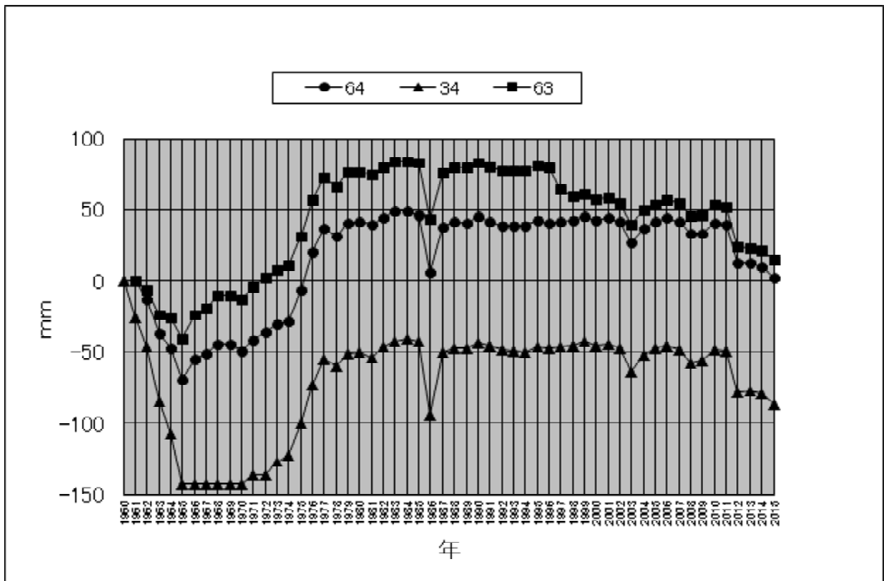
図 2-1-1 鶴見区水準点経年変化
