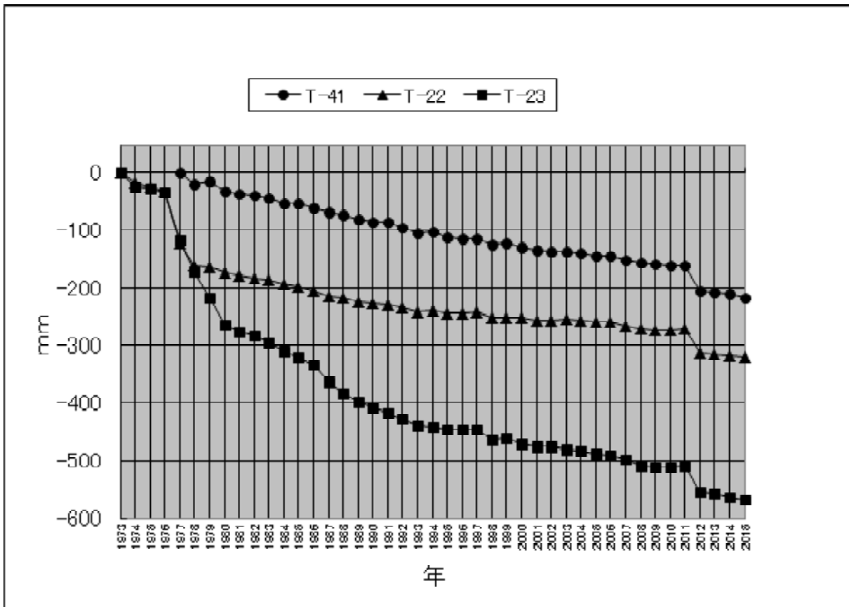
图 2-1-15 戸塚区水準点経年变化
