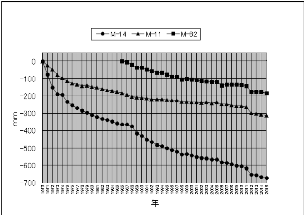
图 2-1-14 都筑区水準点経年变化
