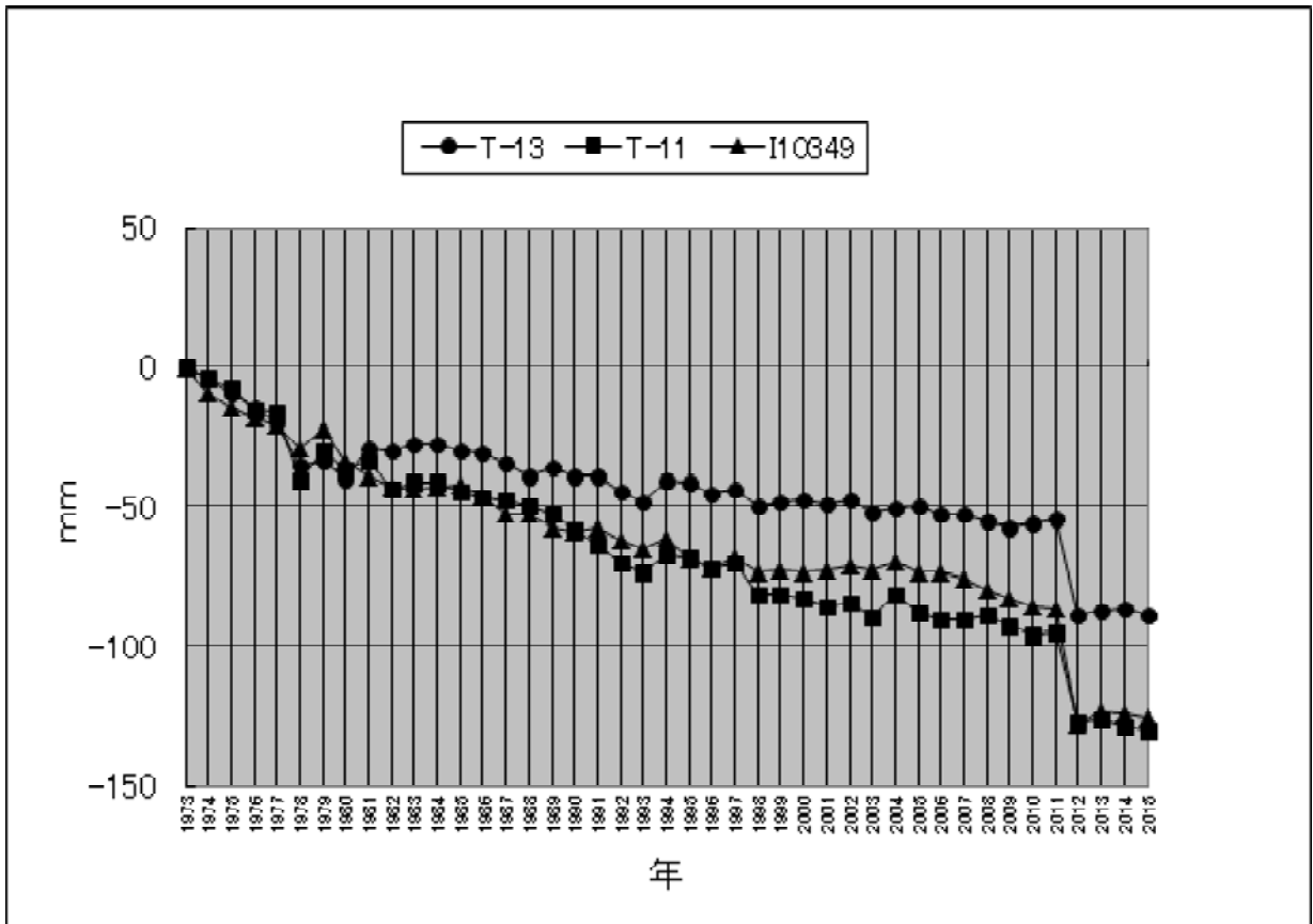
图 2-1-17 泉区水准点经年变化
