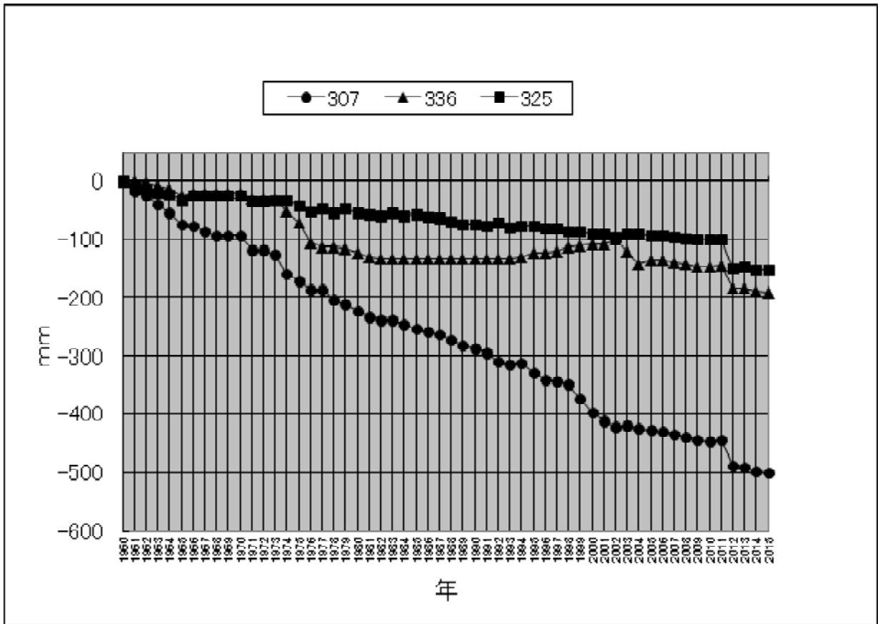
图 2-1-4 中区水準点経年变化
