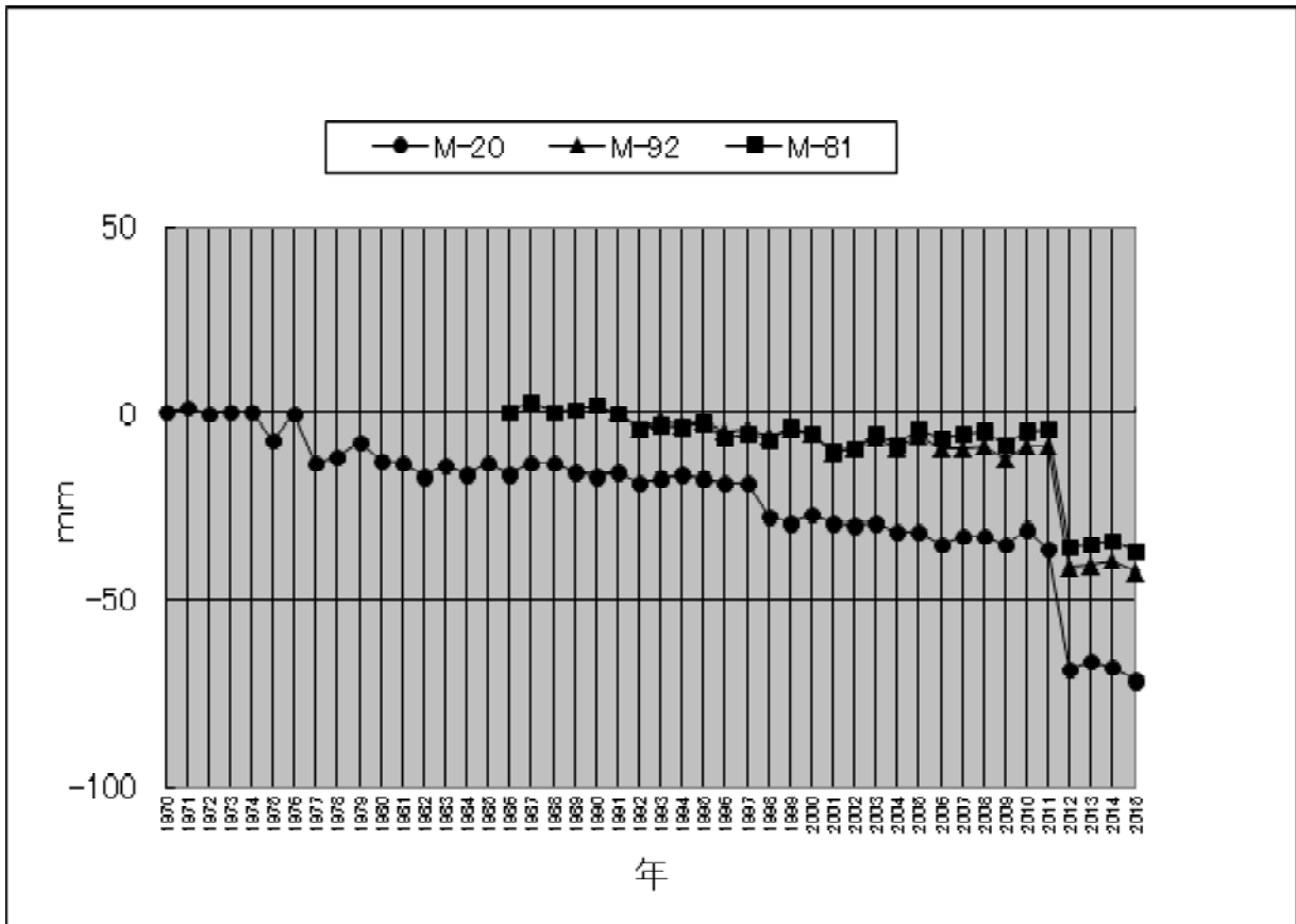
图 2-1-12 緑区水準点経年变化
