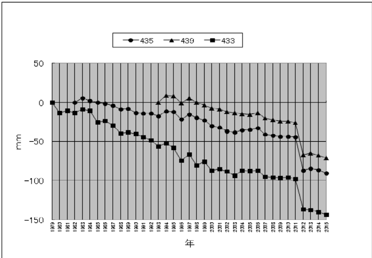
图 2-1-9 磯子区水准点经年变化
