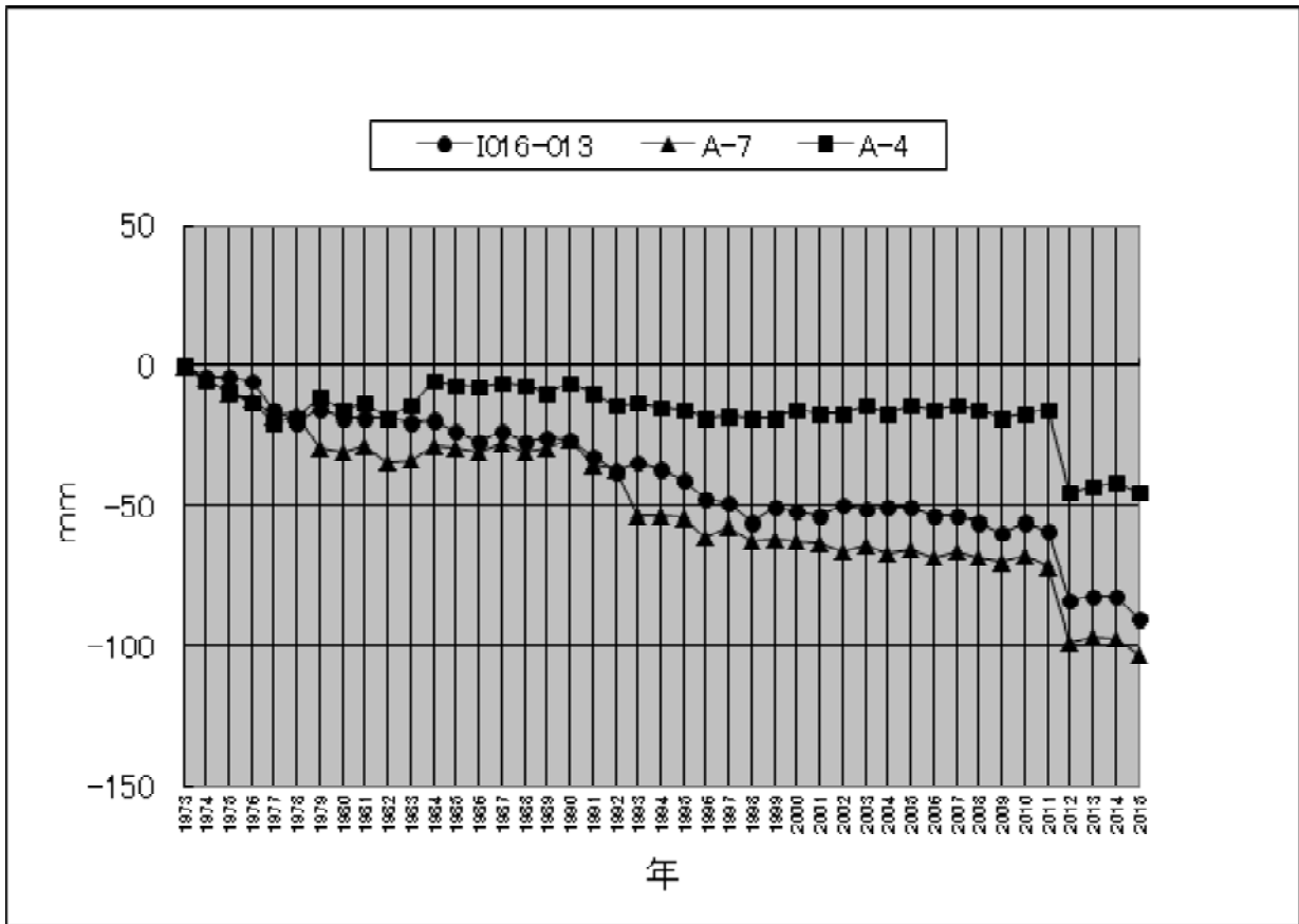
图 2-1-8 旭区水准点经年变化
