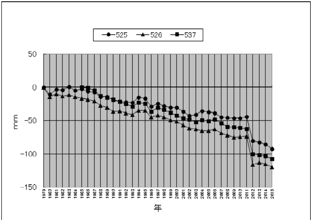
图 2-1-10 金沢区水準点経年变化
