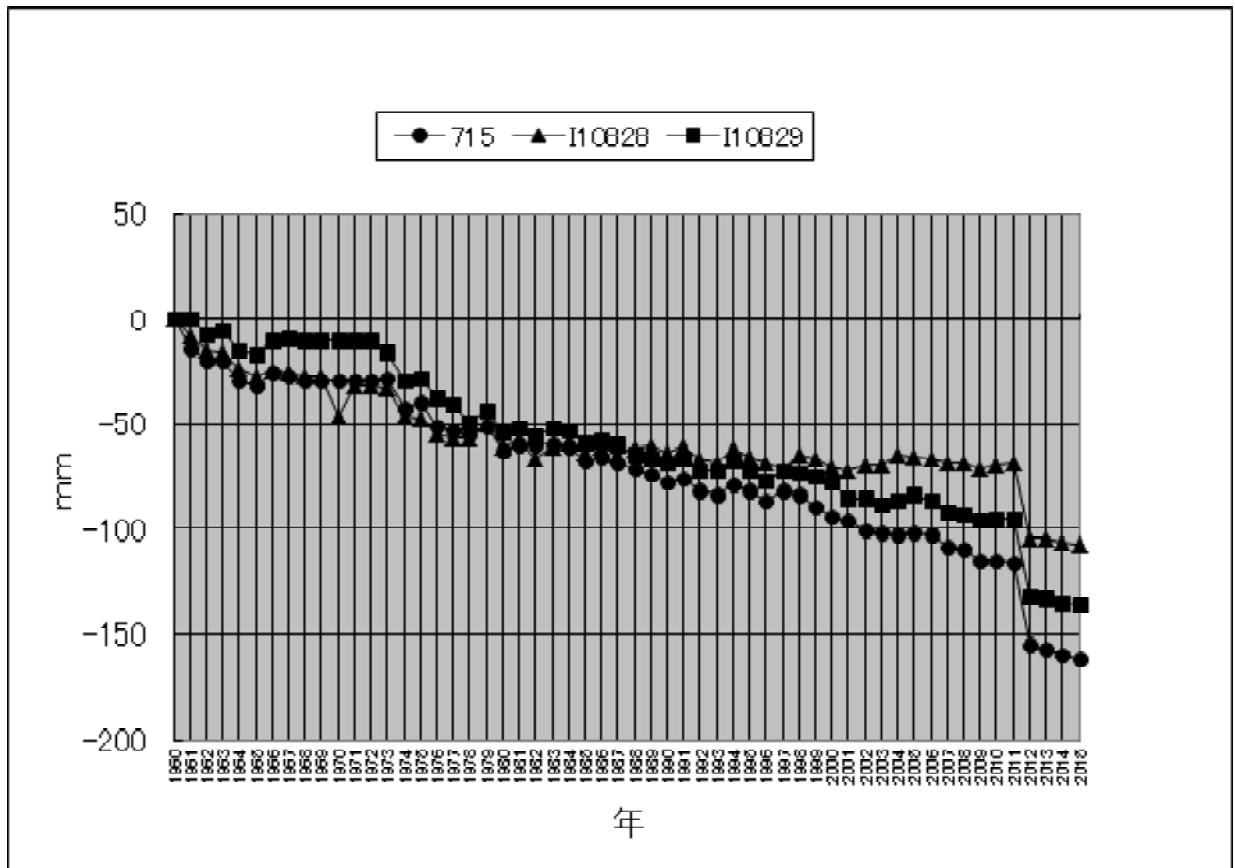
图 2-1-5 南区水準点経年变化
