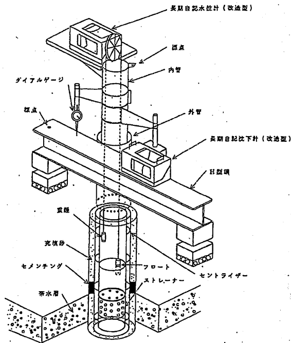
図 2-2-1 地盤沈下観測井戸構造図
