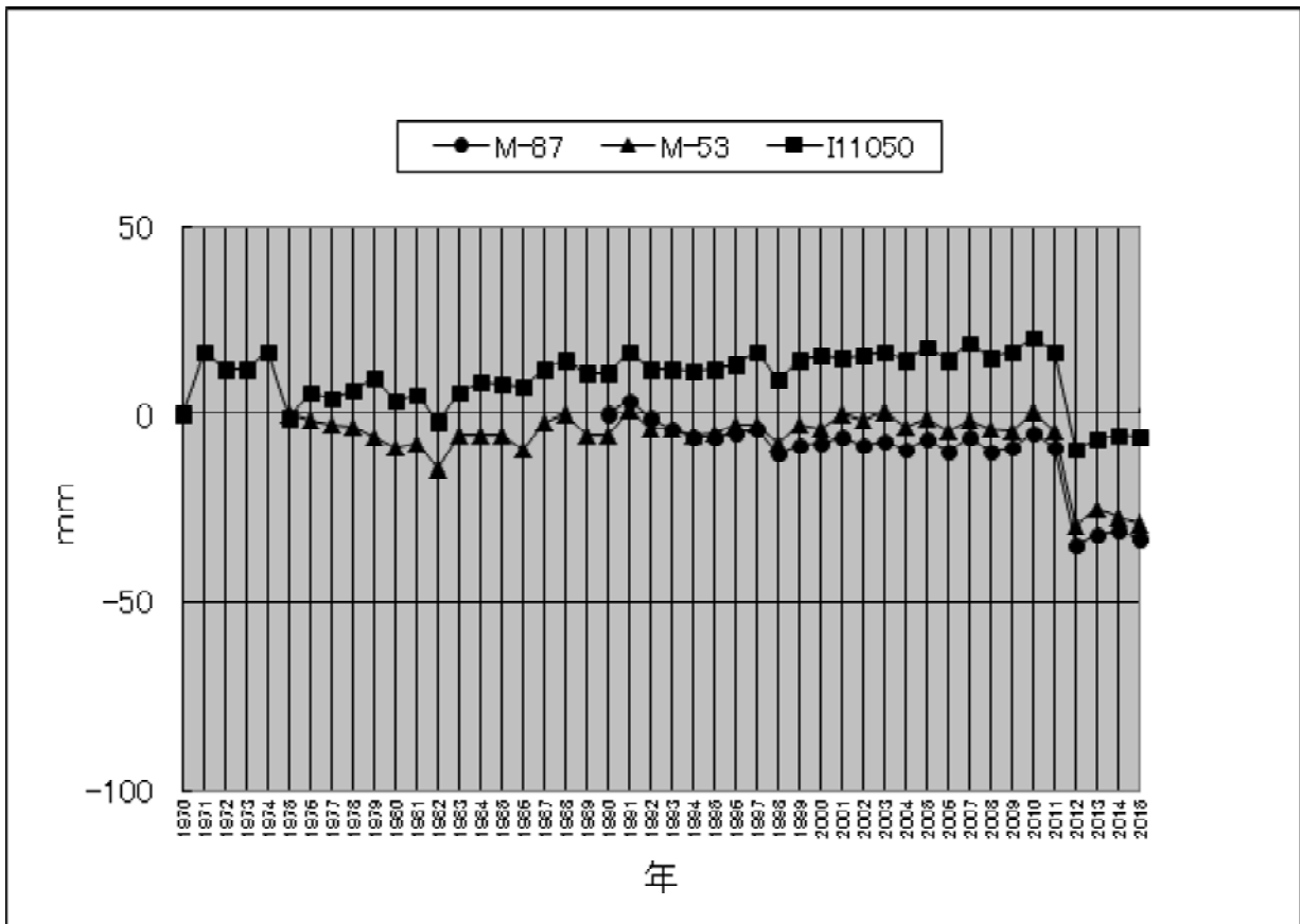
图 2-1-13 青葉区水準点経年变化
