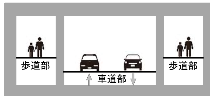
相鉄本線アンダーパス部 ② - ②'
