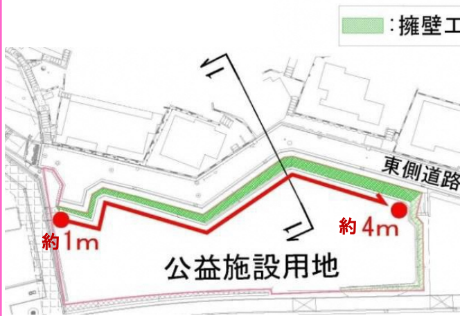
擁壁平面図
