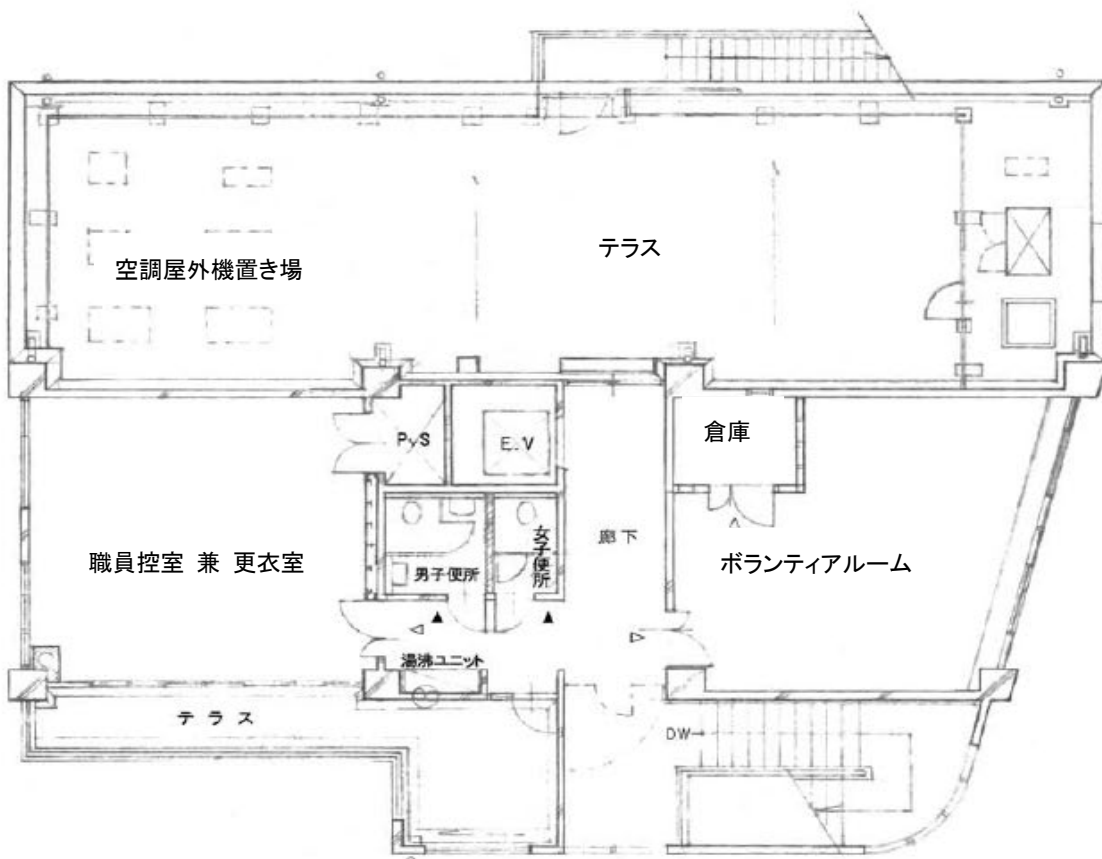
3階 竣工図
