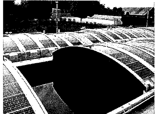
「小雀浄水場ろ過池・ ふくがわい 覆蓋型太陽光発電設備」
