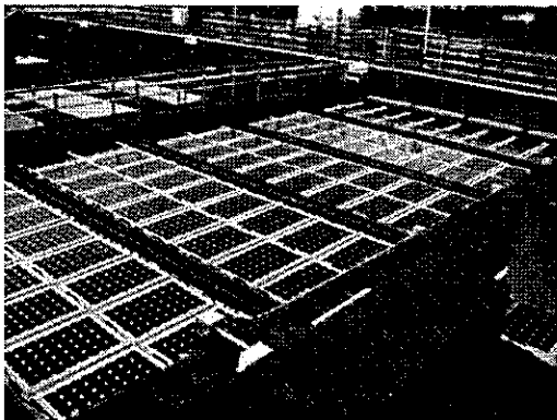
「小雀浄水場沈殿池・フロート型太陽光発電設備」
