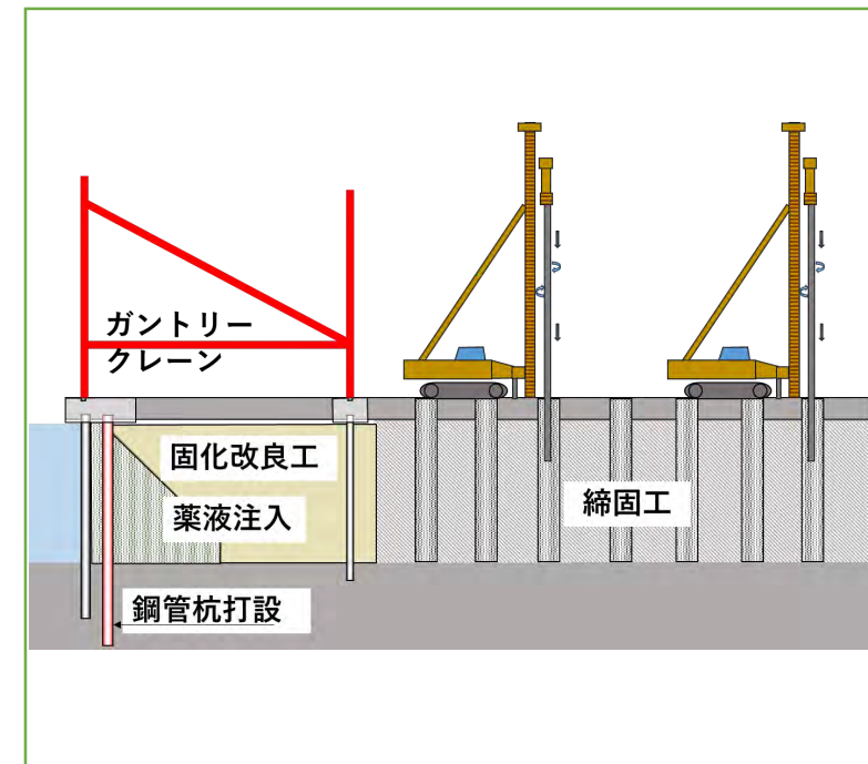
地盤改良概要図
