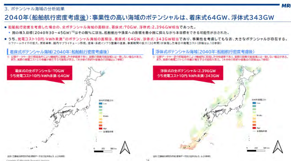
図41 洋上風力のポテンシャル海域分析（株三菱総合研究所報告書より）
