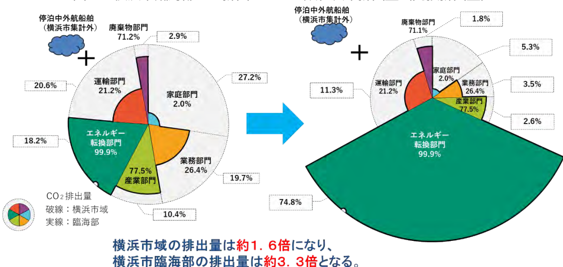
図42 横浜市臨海部から排出される二酸化炭素排出量（間接排出量）
