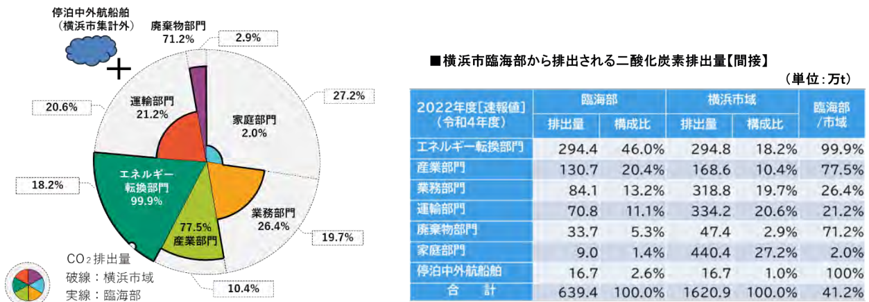
図42 横浜市臨海部から排出される二酸化炭素排出量（間接排出量）
