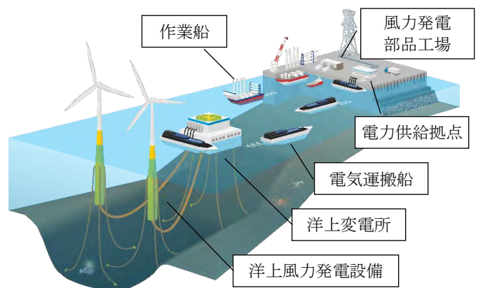
電気運搬船を活用した浮体式洋上風力発電の ウィンドファーム（イメージ）
