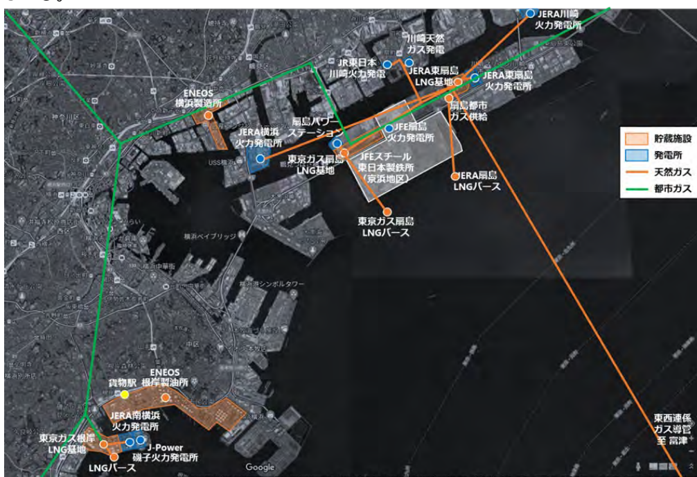
図3 事業用発電所等の既存インフラの立地状況
